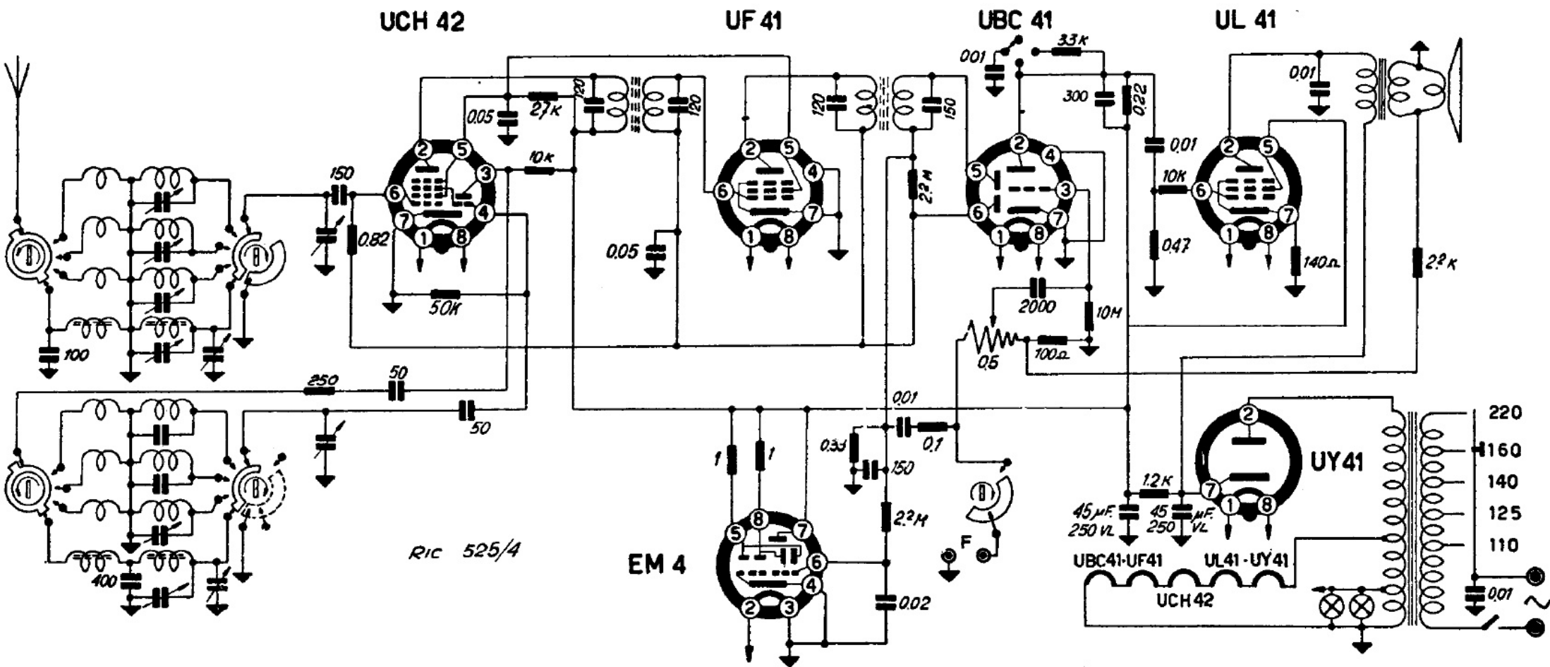
MINERVA RADIO - Mod. Taormina tipo 525/4. Supereterodina con 4 gamme d'onda. Onde medie da 190 a 580 m. Corte da 15,5 a 22,5 m, da 22 a 33,5 m, da 33 a 52 m. Media frequenza 468 kc. Potenza d'uscita 2,5 W. Consumo 40 watt.
